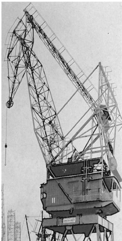
Una delle gru a braccio retrattile costruita dalla Servettaz-Basevi per il porto di Savona.
